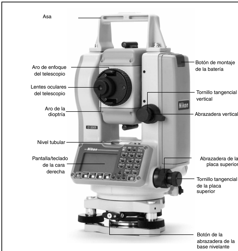
Figura 1.1 Estaciones totales electrónicas de la serie DTM-302 – Cara derecha
